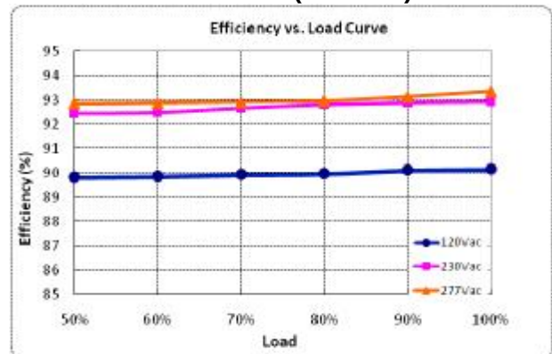
X6-240Y062 (Io=5.71A)
