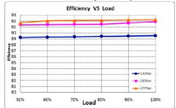
X6-105Y100 (Io=1.40A)
