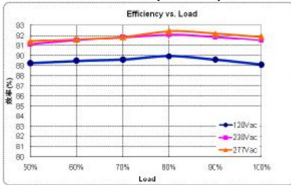
X6-105Y062 (Io=1.69A)
