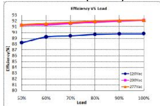
X6-105Y150 (Io=1.05A)
