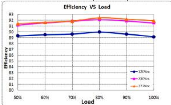
X6-105Y100 (Io=1.05A)
