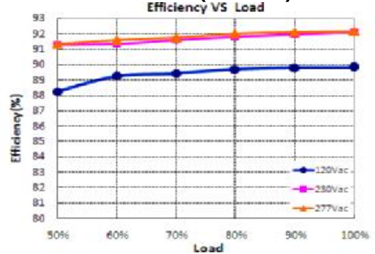
X6-105Y150 (Io=1.05A)
